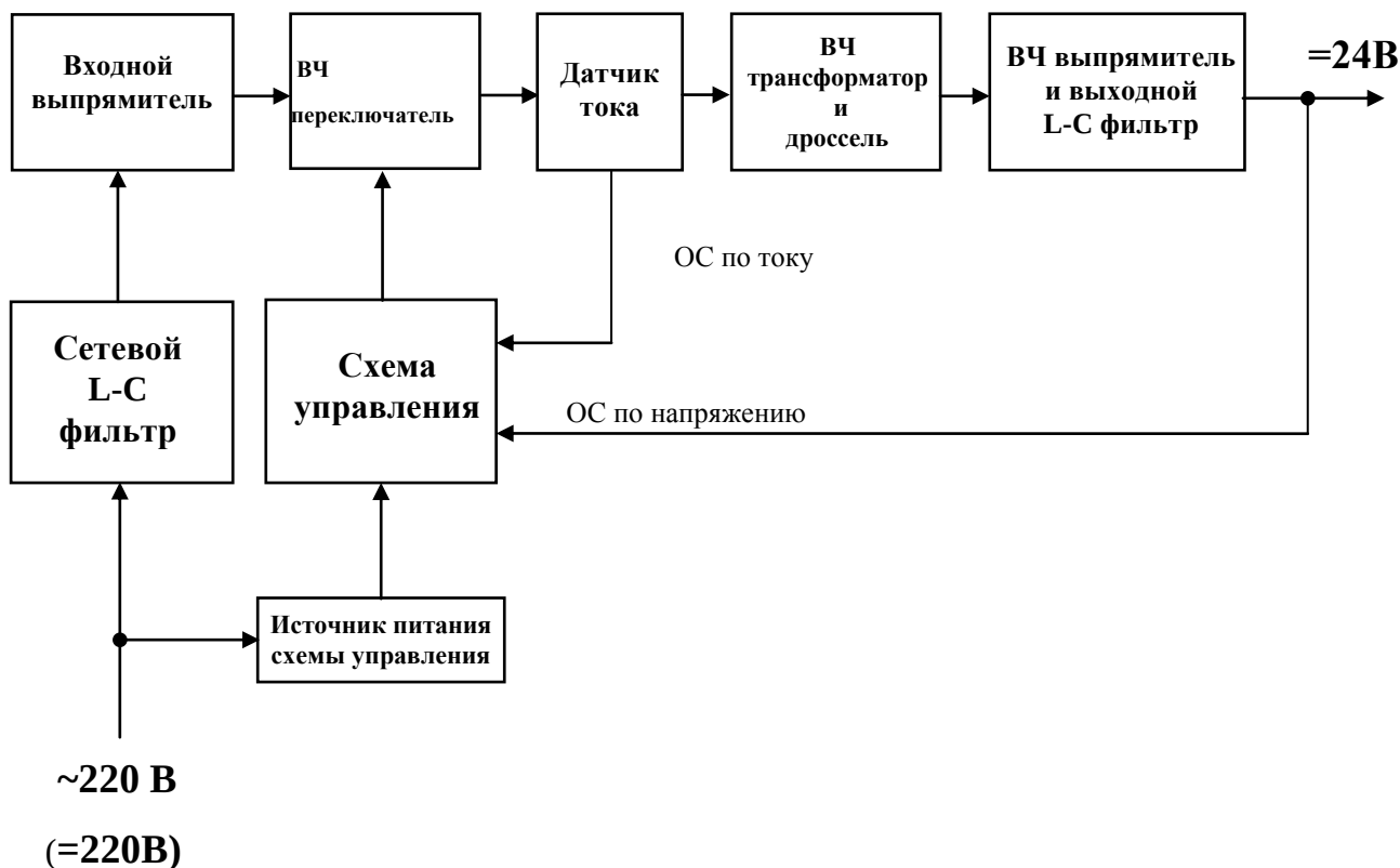
Рис.1. Структурная схема ИПС.
