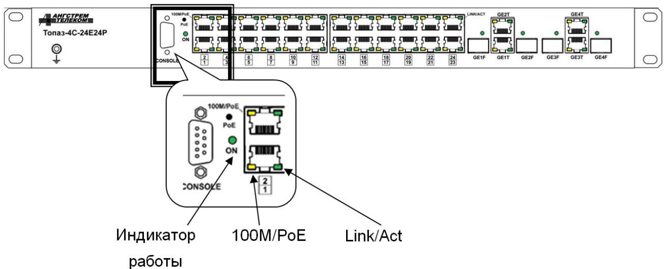
Рисунок 4.3.2 – Элементы индикации и управления коммутаторов в стойку 19'
