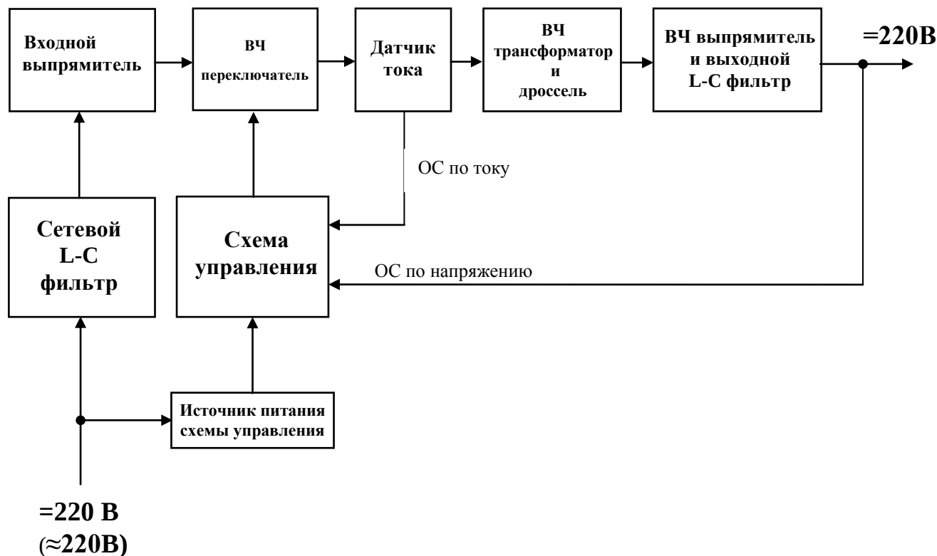
Рис.1. Структурная схема ИПС-300.
