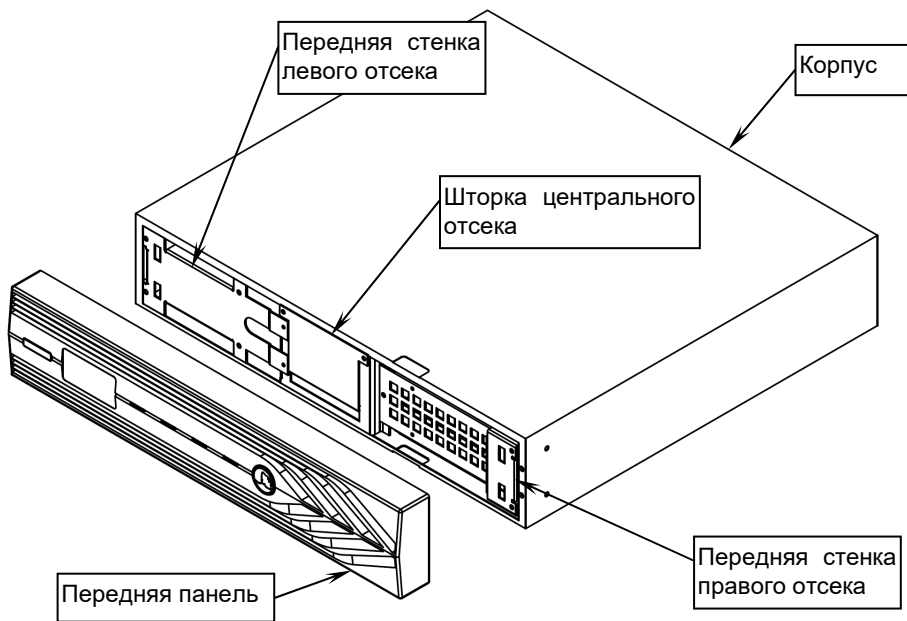
Рисунок 1 – Общий вид ББ со снятой передней панелью
