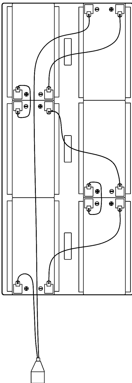
Рисунок 7 — схема соединений АКБ
