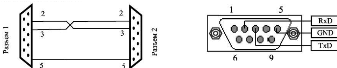
Разъем RS-232. Вилка DB-9M.
