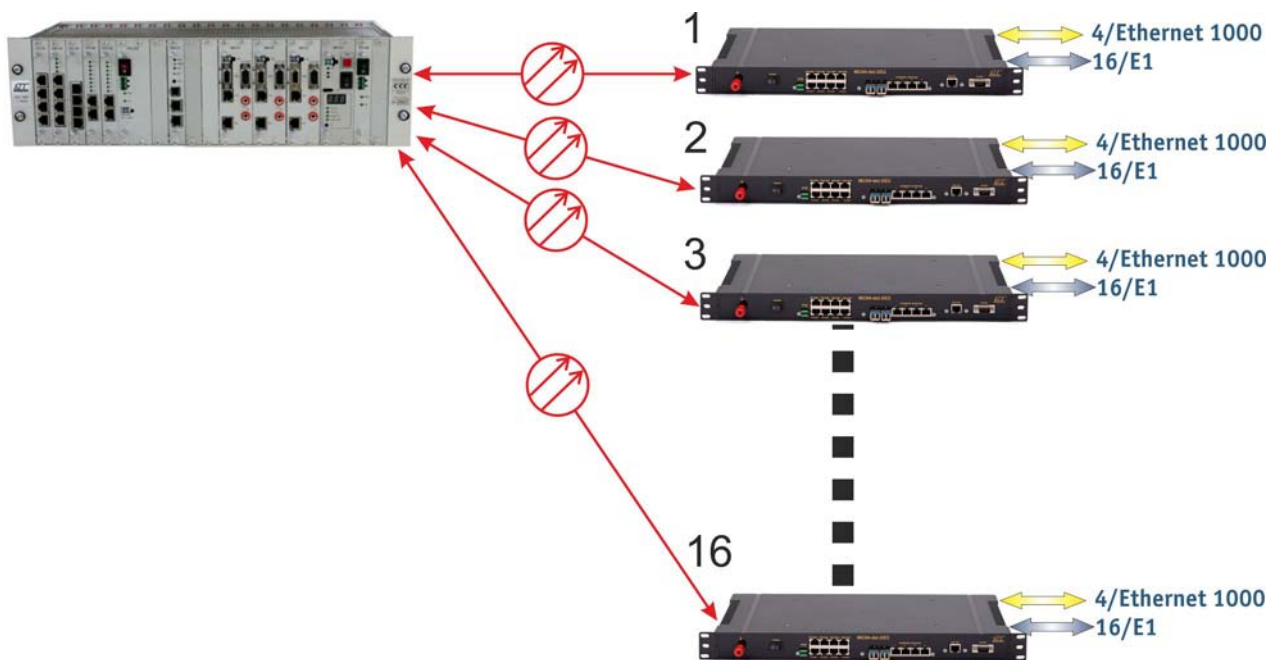
Рис.8 организация связи "звезда" с MC04-DSL-3U
