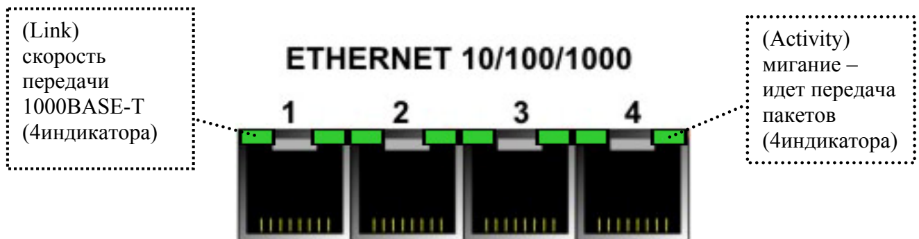
Рис. 11. Разъемы ETHERNET 10/100/1000 модем–мультиплексора MC04– dsl.GE2.
