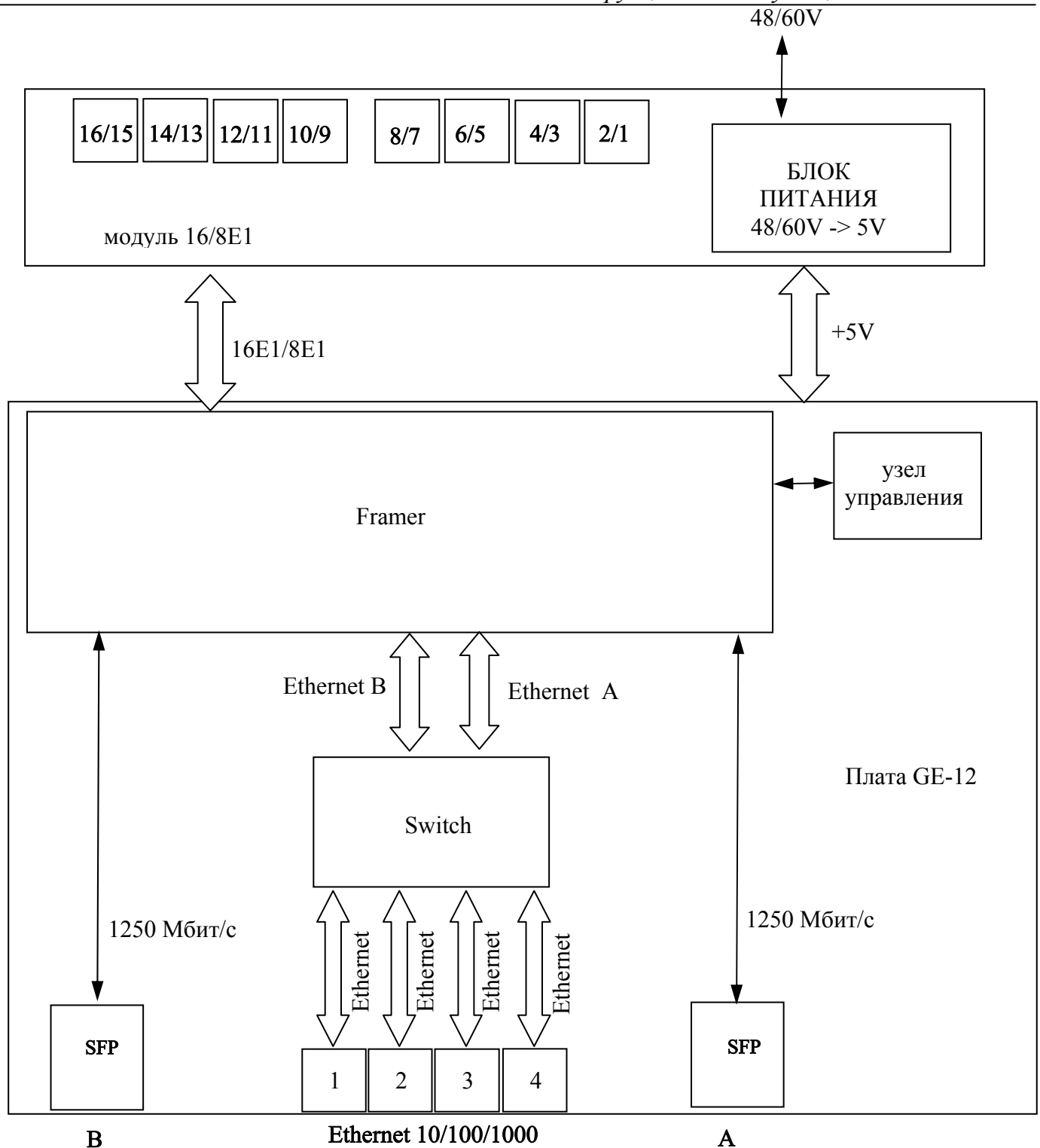
Рис. 10. Блок-схема модема MC04-dsl.GE2.
